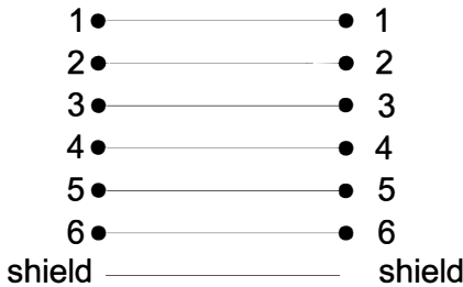
Wiring
