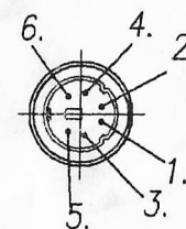
MINI DIN 6M
